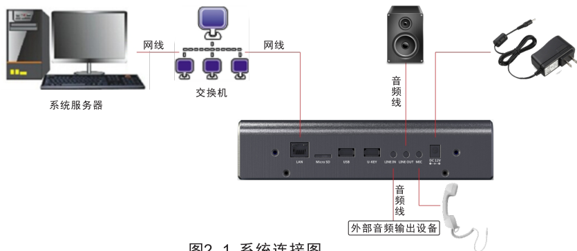
图2.1 系统连接图
